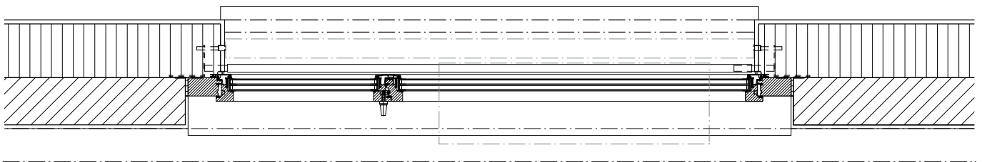
HORIZONTALSCHNITT
