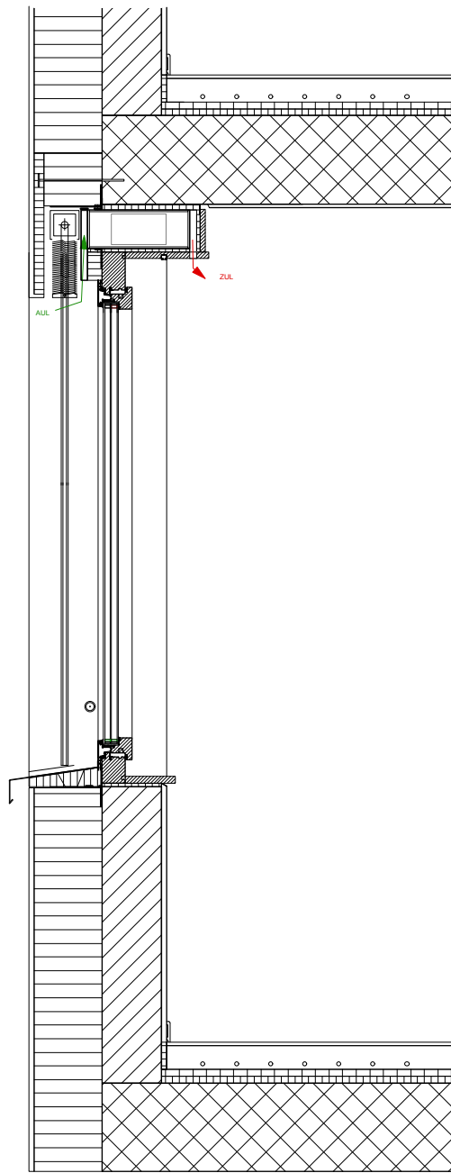
VERTIKALSCHNITT
