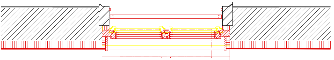
HORIZONTALSCHNITT
